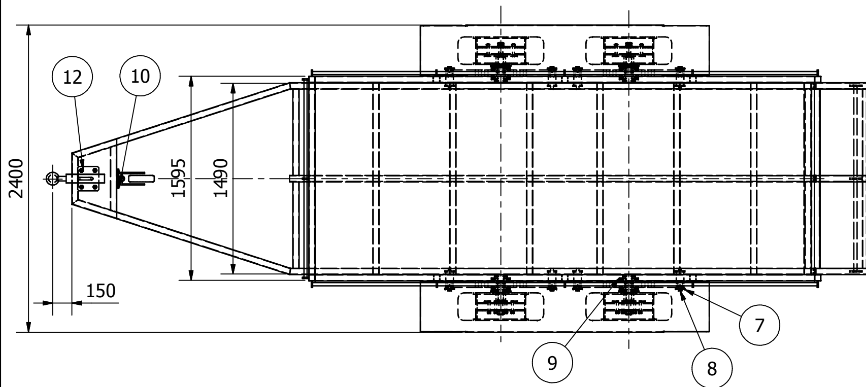
PLAN ( 1 : 30 )
