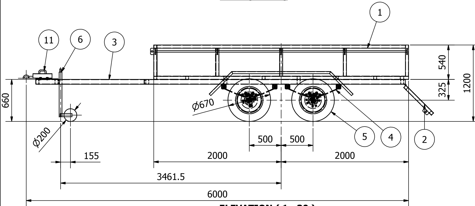
ELEVATION ( 1 : 30 )
