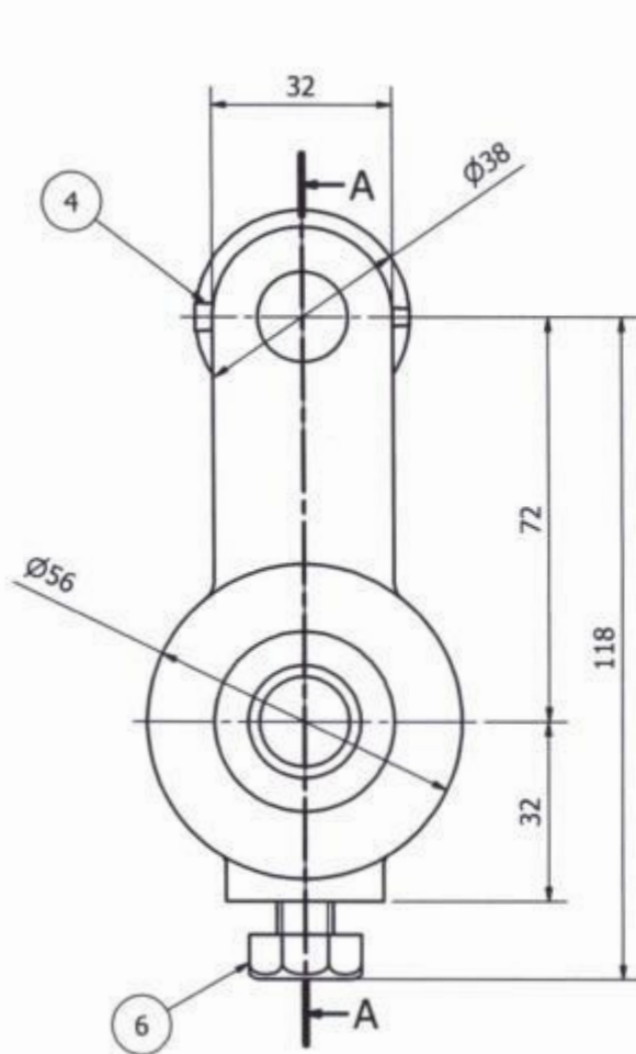
ELEVATION ( 1 : 1 )
