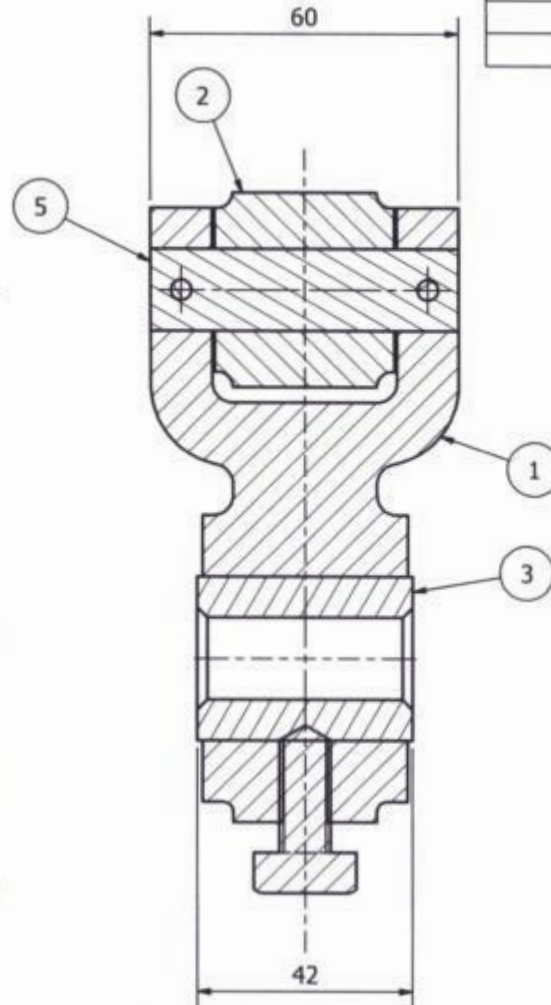
SECTION A-A ( 1 : 1 )
